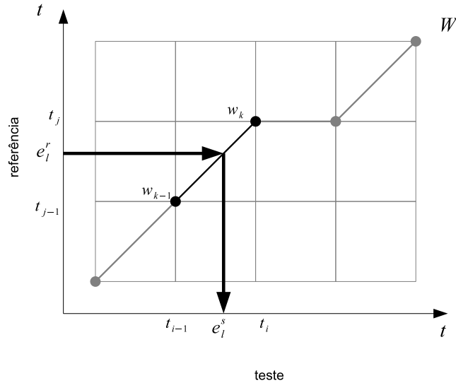
Figura 3.5: Exemplo do mapeamento da etiqueta e_l^r no sinal de referência para a etiqueta e_l^s no sinal de teste, através do caminho de alinhamento W .
